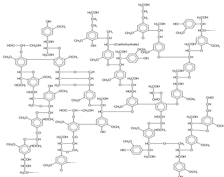
Figure 6: Lignin Structure (Wikimedia Commons 2007c: n.p.)
