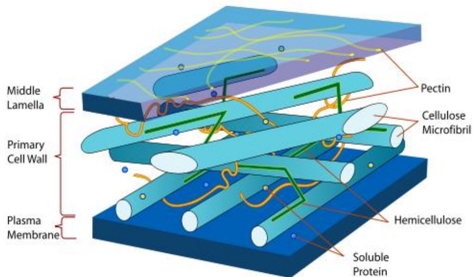
Figure 3: Plant Cell Wall Structure (Wikimedia Commons 2007a: n.p.)
