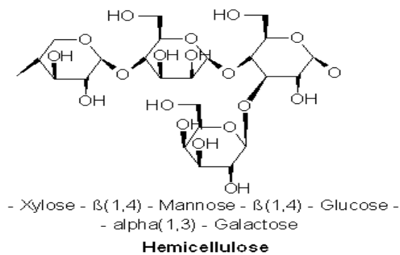
Figure 5: Hemicellulose (Wikimedia Commons 2006: n.p.)
