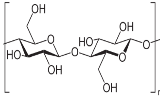
Figure 4: Cellulose (Wikimedia Commons 2007b: n.p.)
