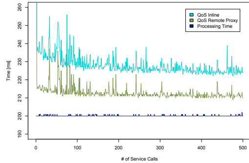
(d) QOS REMOTE PROXY
